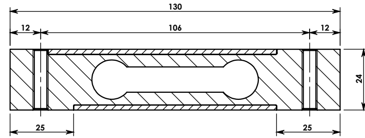
KESIT A-A
