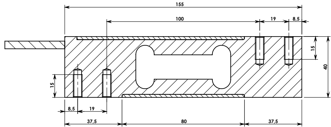
KESİT A-A
