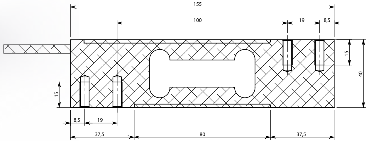
KESIT A-A
