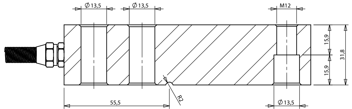
KESİT A-A
